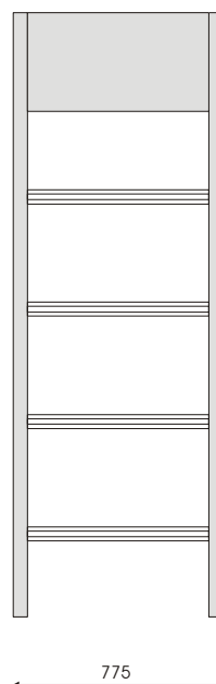
A13175 Torre aperta centrale Dimensioni (mm.) L 775 x P 150 x H 2150
