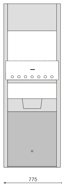
A11075 Torre aperta con vano passante centrale Dimensioni (mm.) L 775 x P 150 x H 2150
