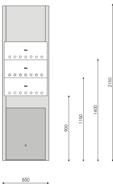
A18165 Torre chiusa a parete Dimensioni (mm.) L 650 x P 150 x H 2150
