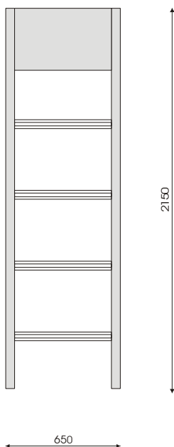
A12165 Torre aperta a parete Dimensioni (mm.) L 650 x P 150 x H 2150
