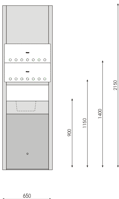
A10165 Torre chiusa con vano passante a parete Dimensioni (mm.) L 650 x P 150 x H 2150
