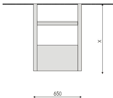
A12065 Supporto a soffitto parete Dimensioni (mm.) L 650 x P 150 x H x = variabile
