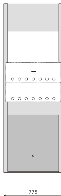
A19075 Torre aperta 2 livelli centrale Dimensioni (mm.) L 775 x P 150 x H 2150
