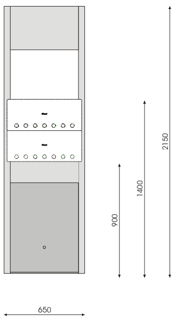
A18065 Torre aperta 2 livelli a parete Dimensioni (mm.) L 650 x P 150 x H 2150
