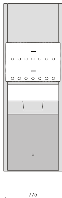
A11175 Torre chiusa con vano passante centrale Dimensioni (mm.) L 775 x P 150 x H 2150
