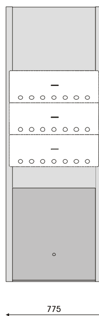
A19175 Torre chiusa centrale Dimensioni (mm.) L 775 x P 150 x H 2150
