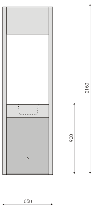
A14065 Torre aperta a parete senza alzata Dimensioni (mm.) L 650 x P 150 x H 2150
