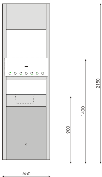
A10065 Torre aperta con vano passante a parete Dimensioni (mm.) L 650 x P 150 x H 2150
