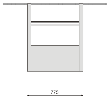
A13075 Supporto a soffitto centrale Dimensioni (mm.) L 775 x P 150 x H x = variabile
