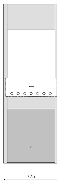
A17075 Torre aperta 1 livello centrale Dimensioni (mm.) L 775 x P 150 x H 2150
