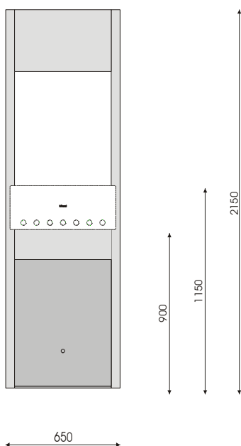
A16065 Torre aperta 1 livello a parete Dimensioni (mm.) L 650 x P 150 x H 2150
